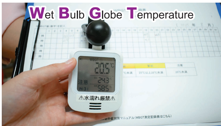
WBGT指数計：上部の黒球によって放射熱(日射や照り返し)を測定できる
